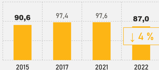
Sunaudotos šilumos energijos kiekis Savivaldybės BĮ pastatuose, kW/m²
